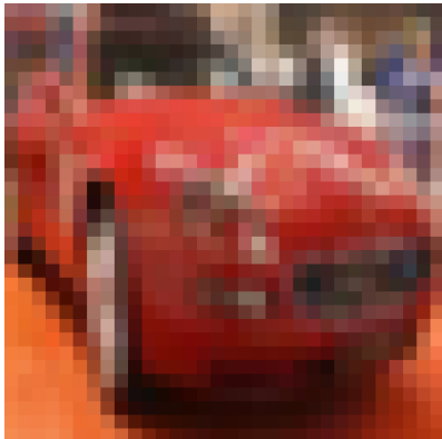
Automobile
